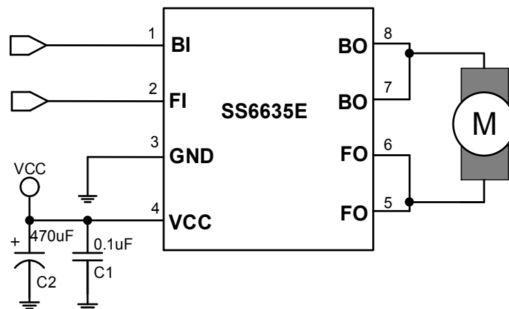
图 1. 典型应用原理图
